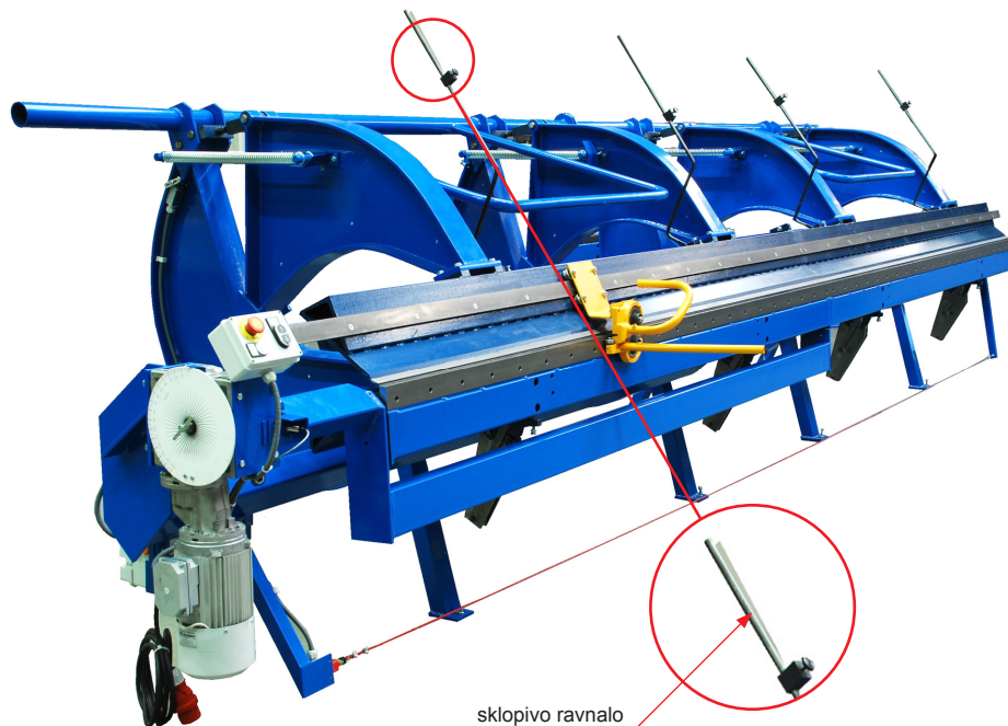
sklopivo ravnalo
